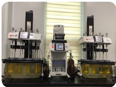
용출시험기
